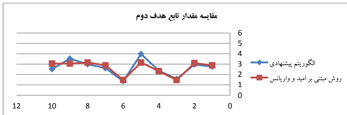
شکل ۲. مقایسه مقادیر پارتنوی تابع هدف Z^{(2)}
