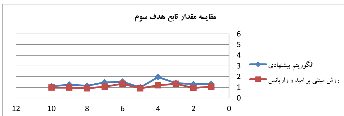
شکل ۳. مقایسه مقادیر پارتنوی تابع هدف Z^{(3)}
